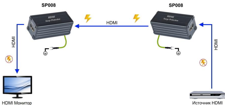
Рис.2 Схема подключения SP008
