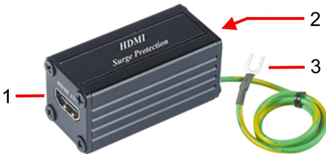
Рис.1 Внешний вид устройства SP008, разъемы подключения
